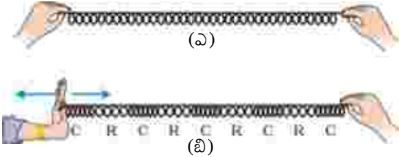
పటం 11.5: స్ప్రింగ్ లో అనుదైర్ఘ్య తరంగాలు
