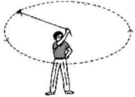
పటం 9.1: స్థిర పరిమాణం గల వేగంతో వృత్తాకార మార్గంలో చలిస్తున్న రాయి గురించి వర్ణించుట.
