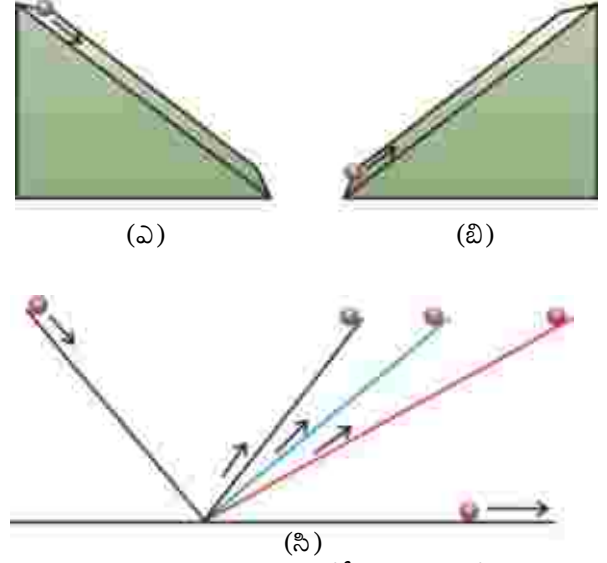
పటం 8.5: (ఎ) వాలుతలంపై గోళీ యొక్క అభ్రోచలనం (బి) వాలుతలంపై గోళీ యొక్క ఊర్జ్వచలనం (సి) రెండువైపులా వాలు గల తలం మీద
