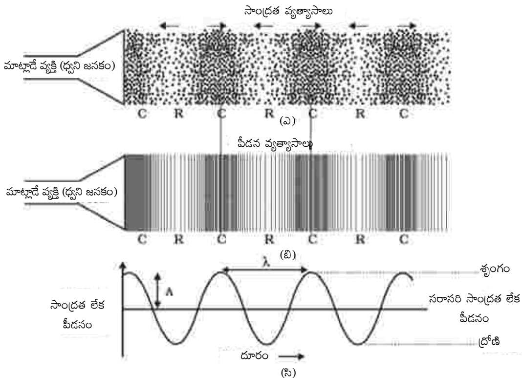
పటం 11.6: (ఎ), (బి) లో చూపినవిధంగా సాంద్రత లేదా పీడన వ్యత్యాసాలతో ధ్వని ప్రయాణించుట, సాంద్రత మరియు పీడన వ్యత్యాసాలను పటం (సి) లో గ్రాఫ్ రూపంలో చూపబడ్డాయి.
